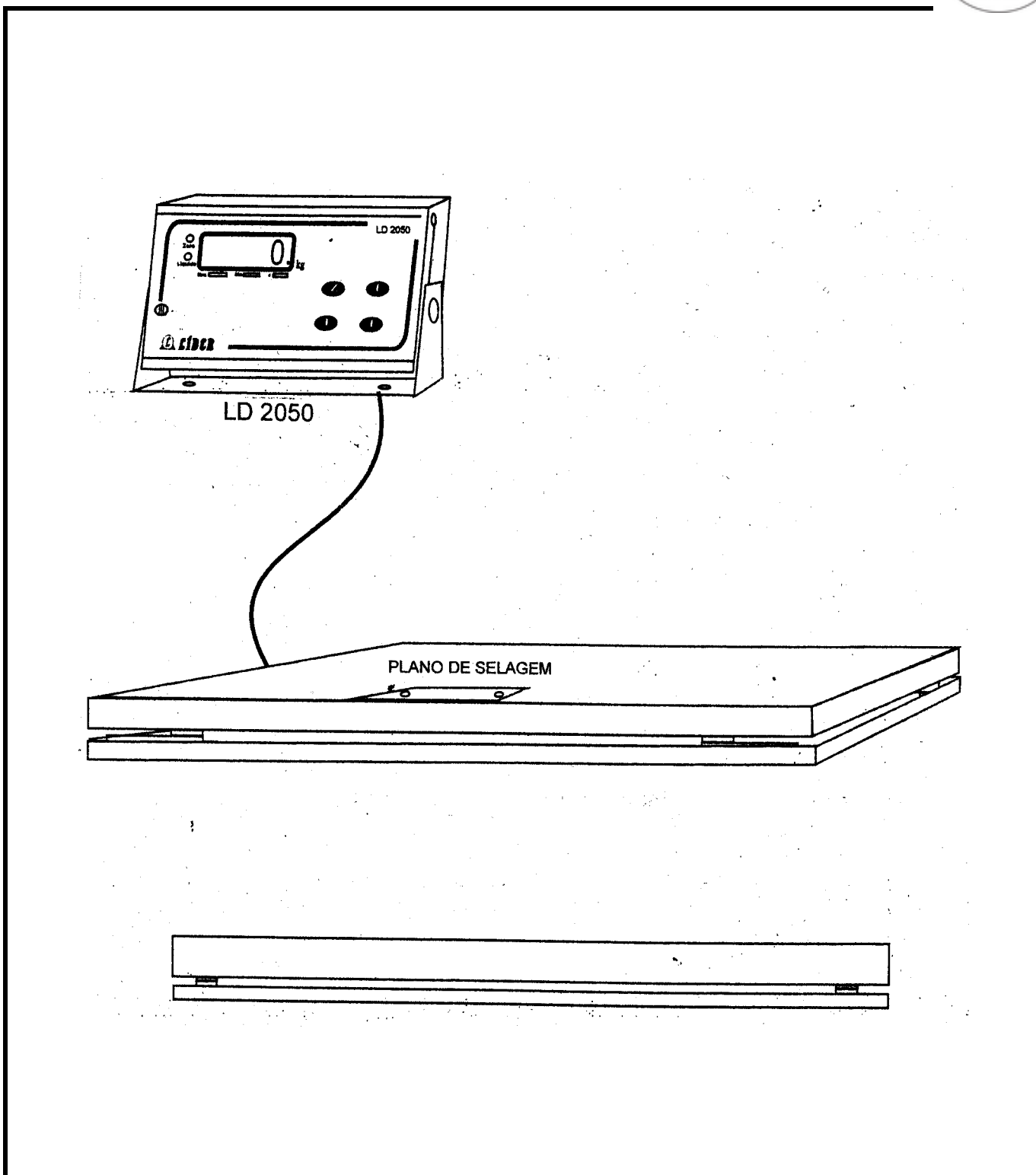
DESENHO ANEXO À PORTARIA INMETRO/DIMEL N° 232, DE 08 DE agosto DE 2008.
