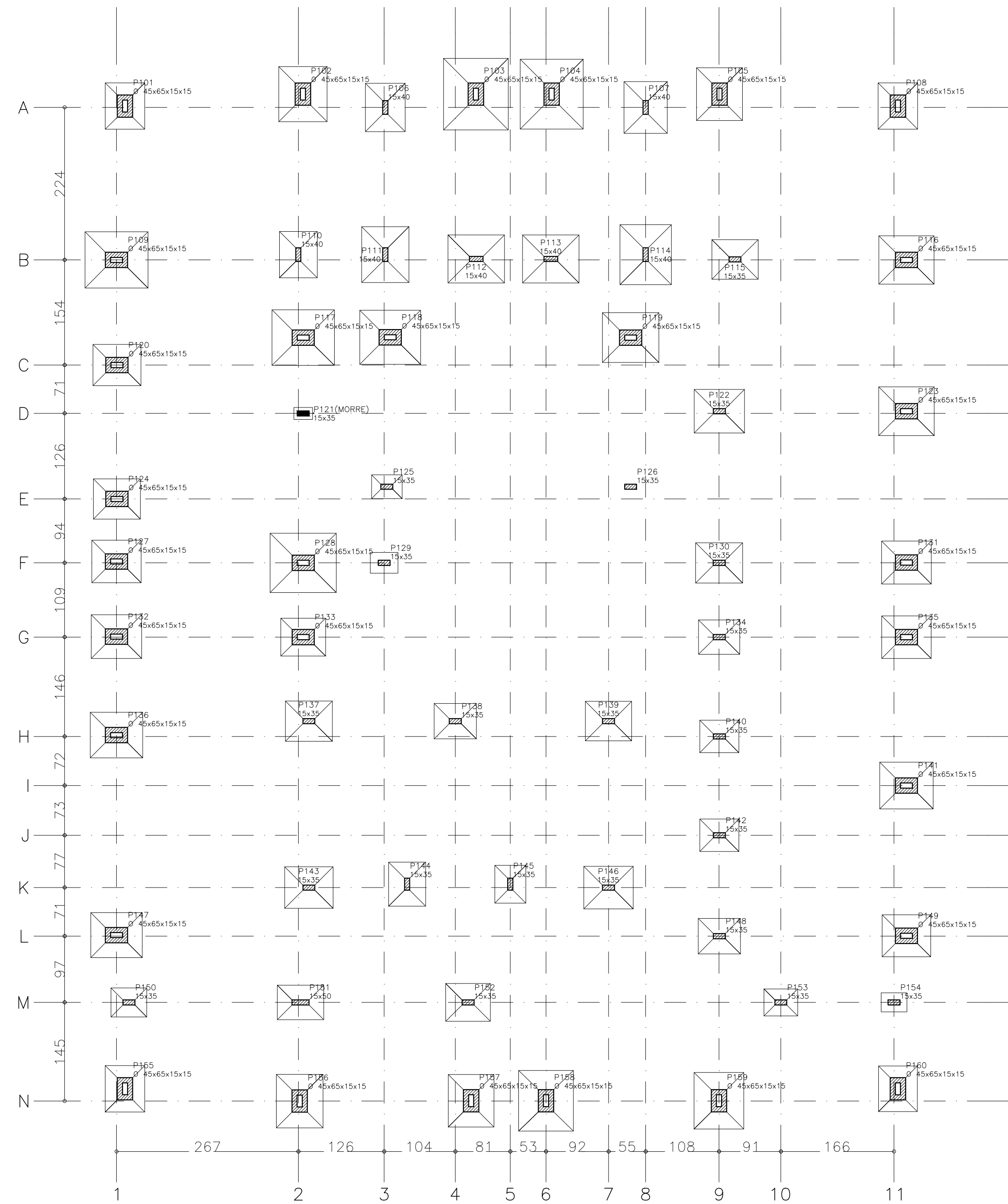
FORMA DO PAVIMENTO BALDRAME ESC.: 1:100
