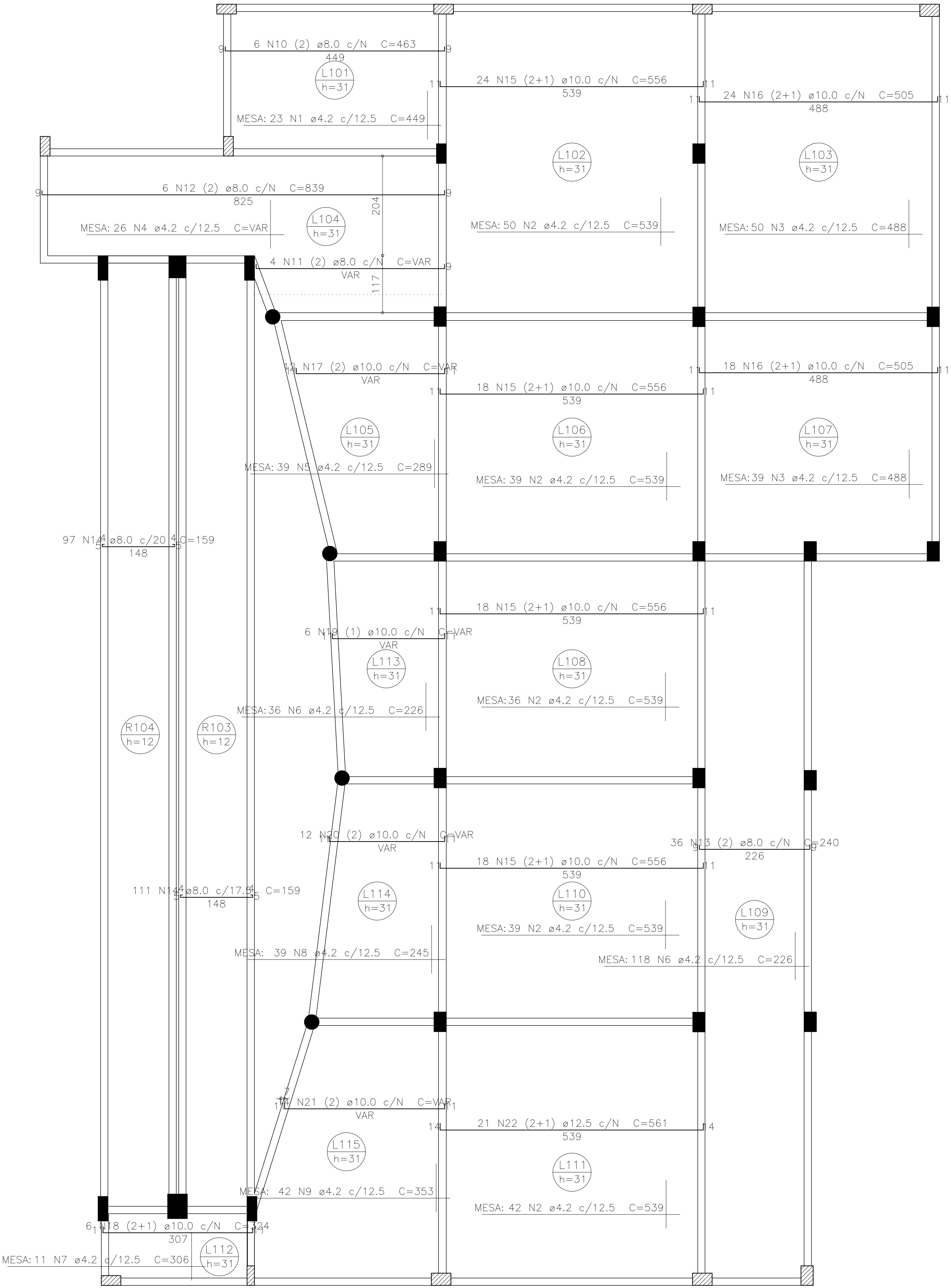
ARMAÇÃO POSITIVA – LAJES 2° PAVTO (EIXO X) ESC.: 1:50
