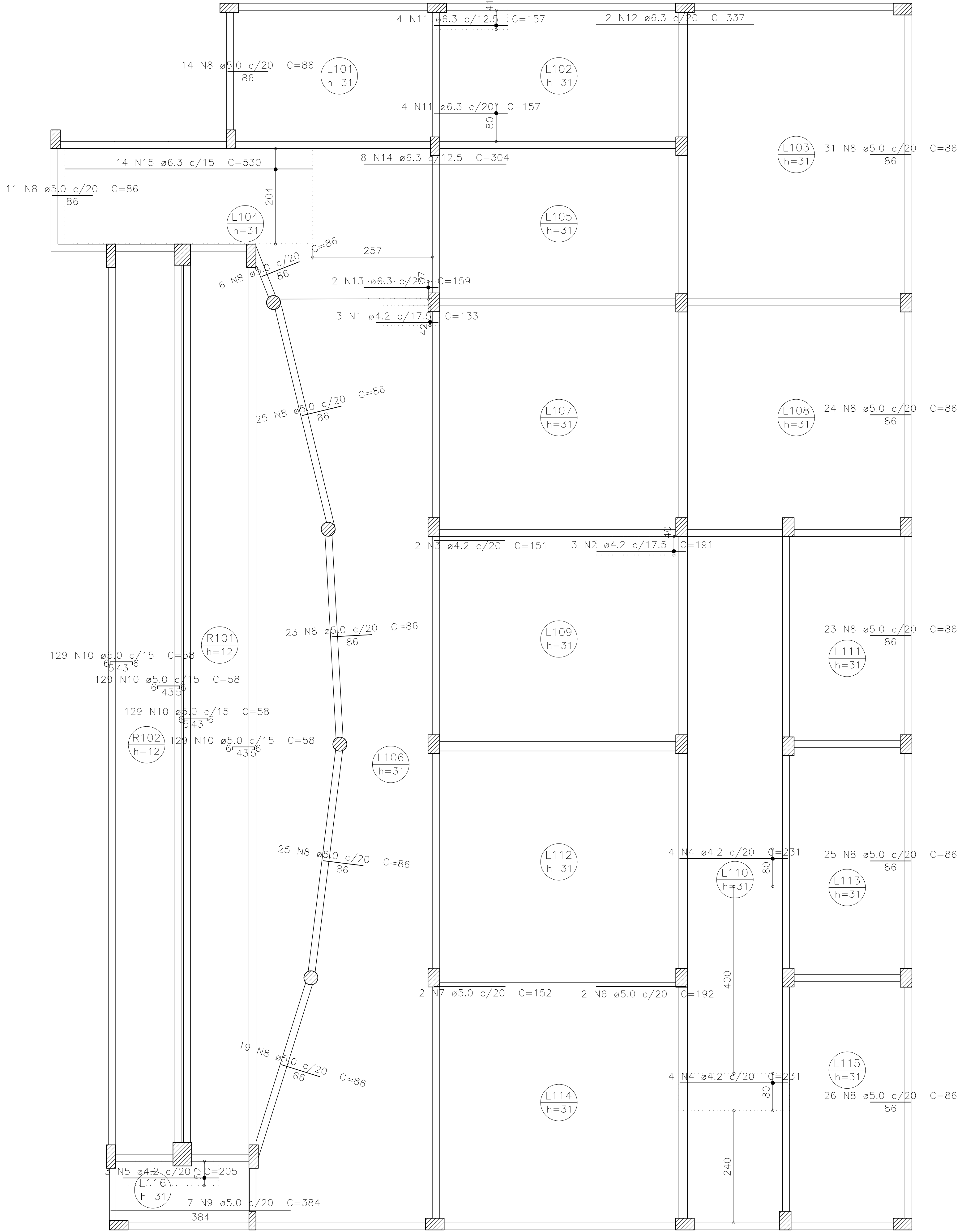
ARMAÇÃO NEGATIVA – LAJES 1º PAVTO (EIXO X) ESC.: 1:50
