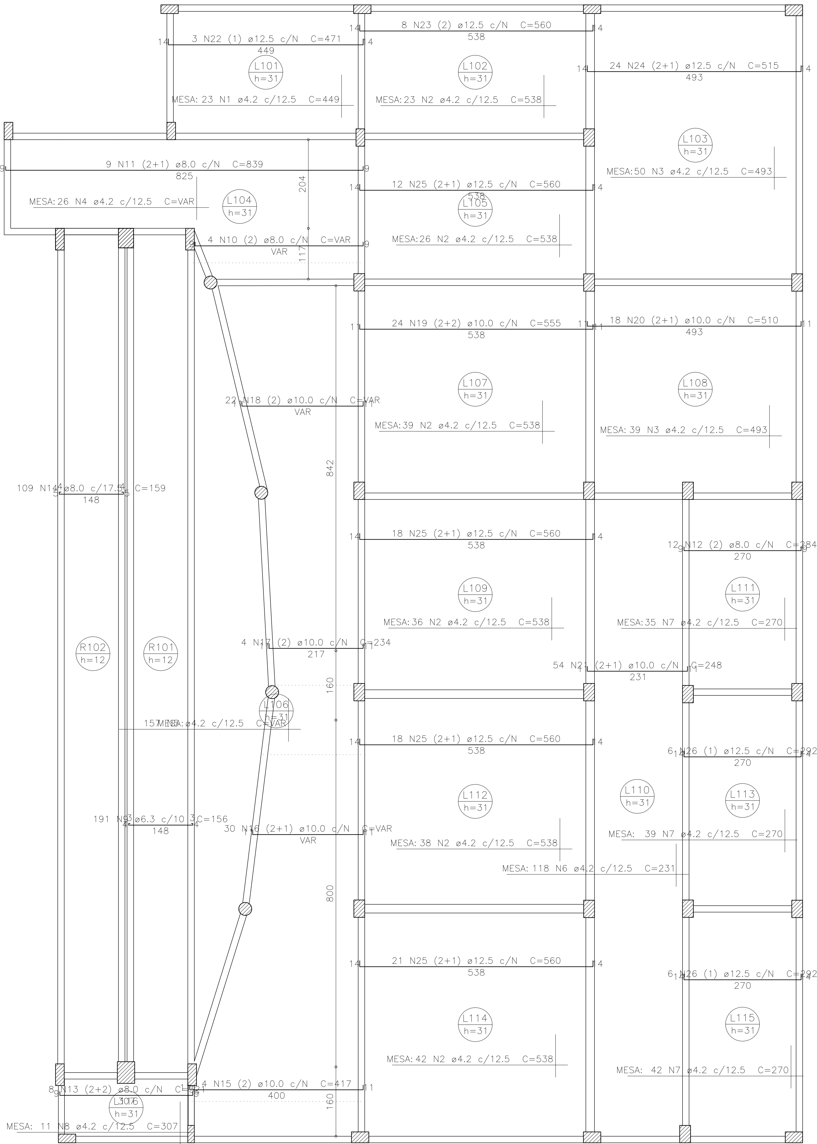
ARMAÇÃO POSITIVA – LAJES 1º PAVTO (EIXO X) ESC.: 1:50
