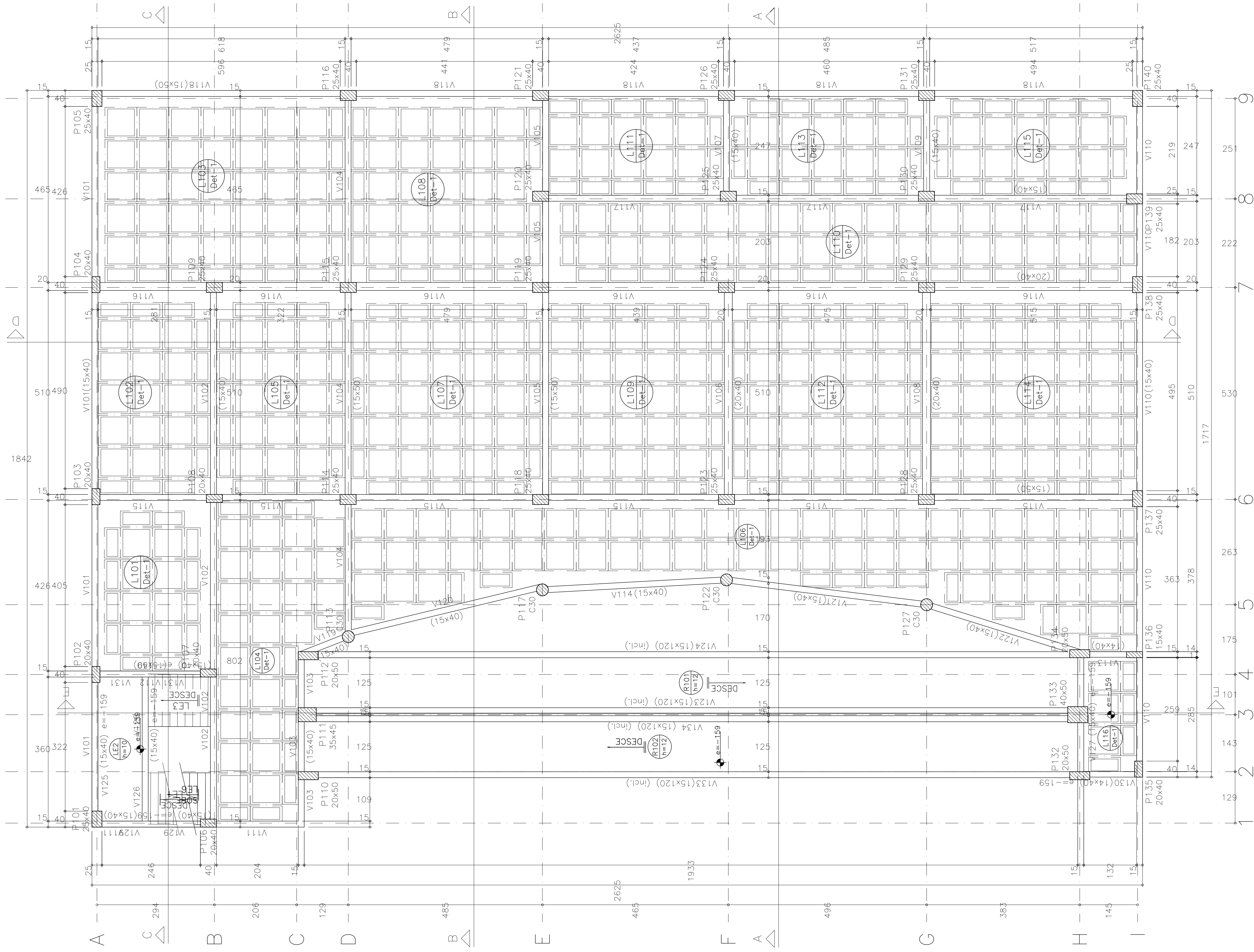
FORMA – 1º PAVTO (NÍVEL 349) ESC.: 1:50
