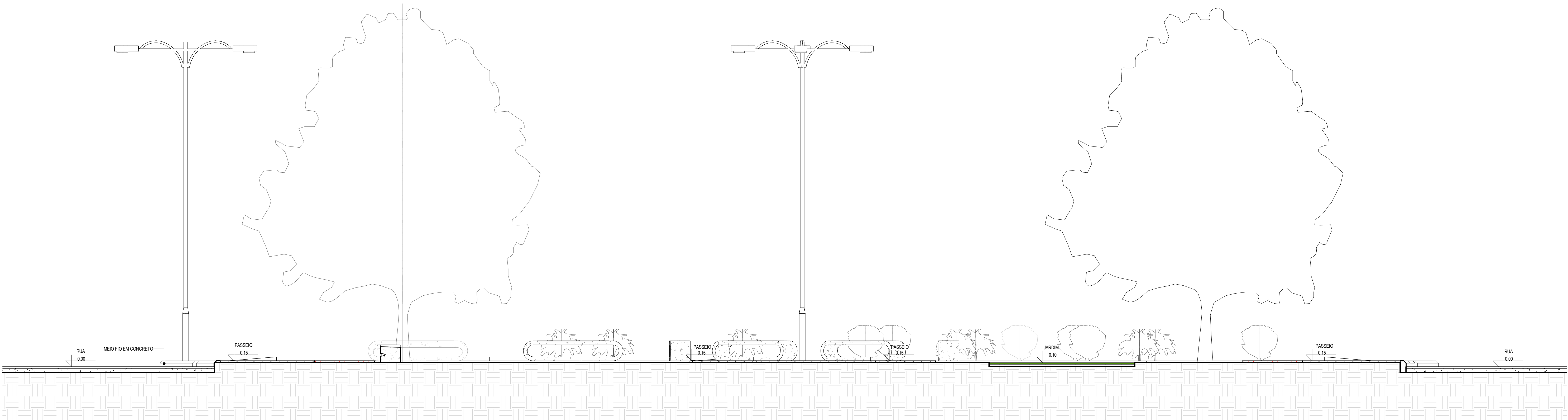
1 CORTE A-A ESCALA 1:50
