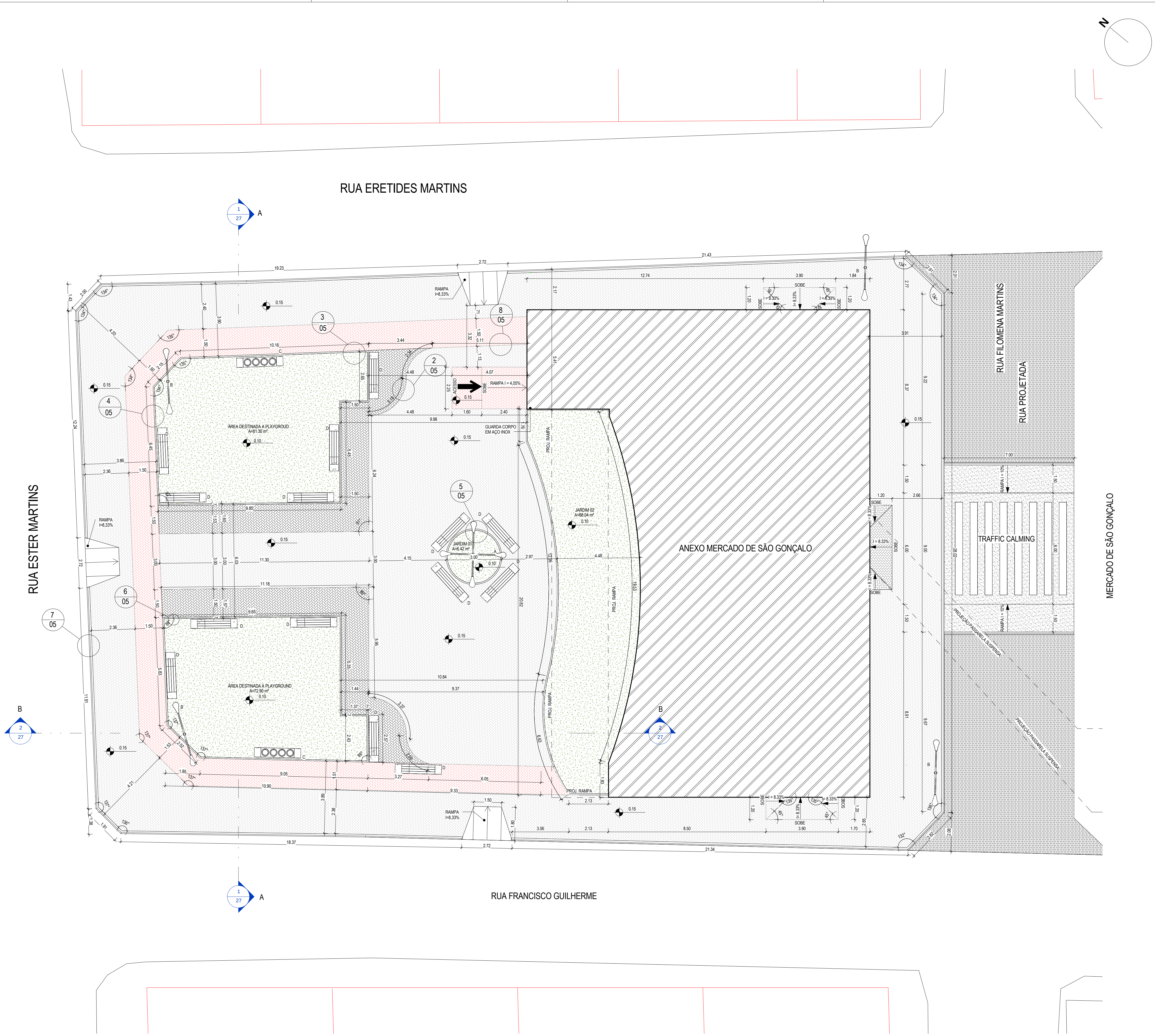
1 PLANTA TÉCNICA ESCALA 1 : 100
