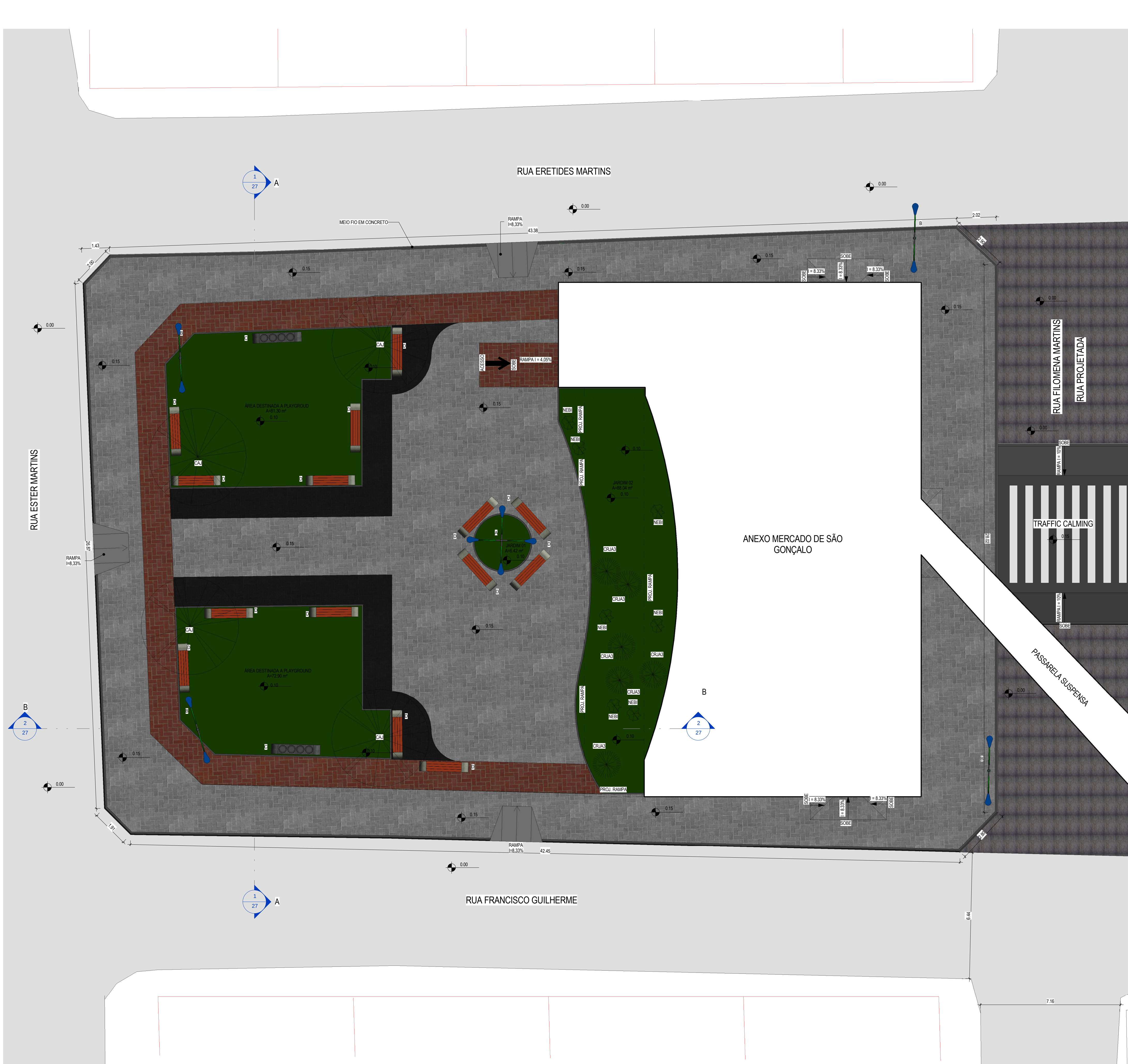
1 PLANTA DE URBANIZAÇÃO / PAISAGISMO ESCALA 1 : 100
