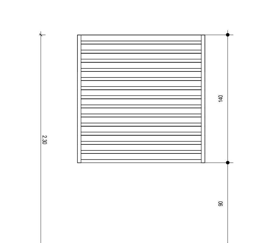
J01 ELEVÇÃO 1/25
