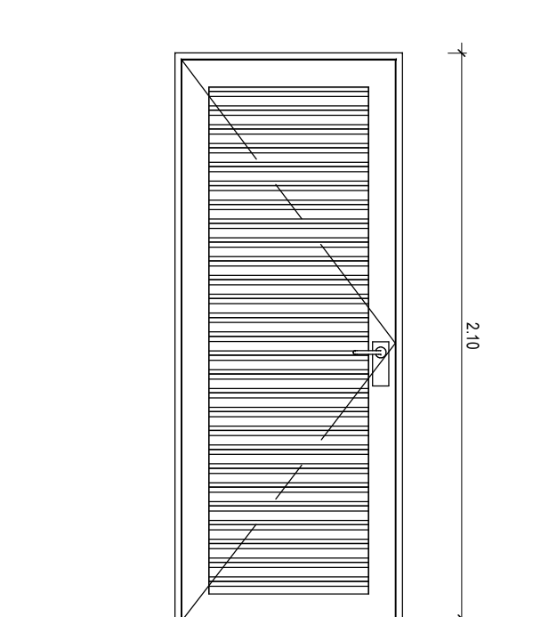
P10 ELEVÇÃO 1/25
