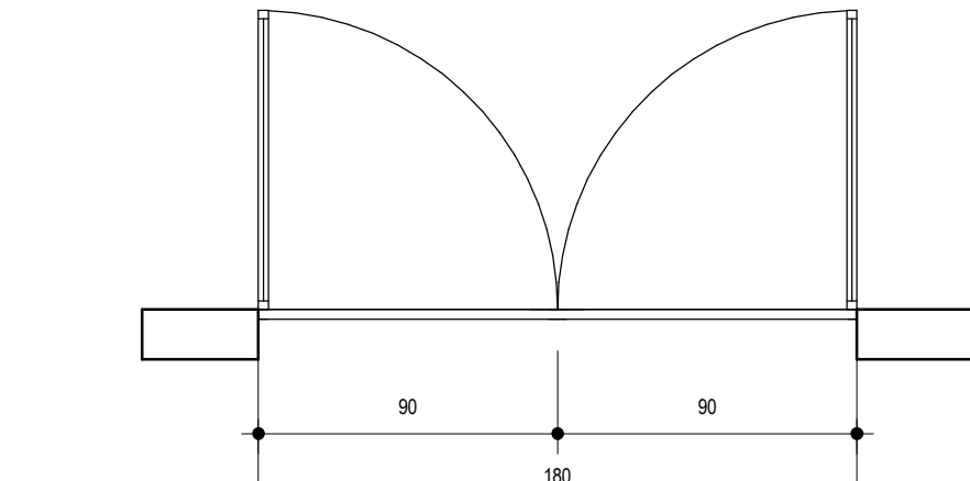
P07 PLANTA 1/25
