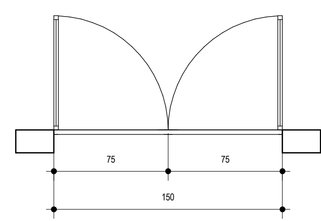
P08 PLANTA 1/25
