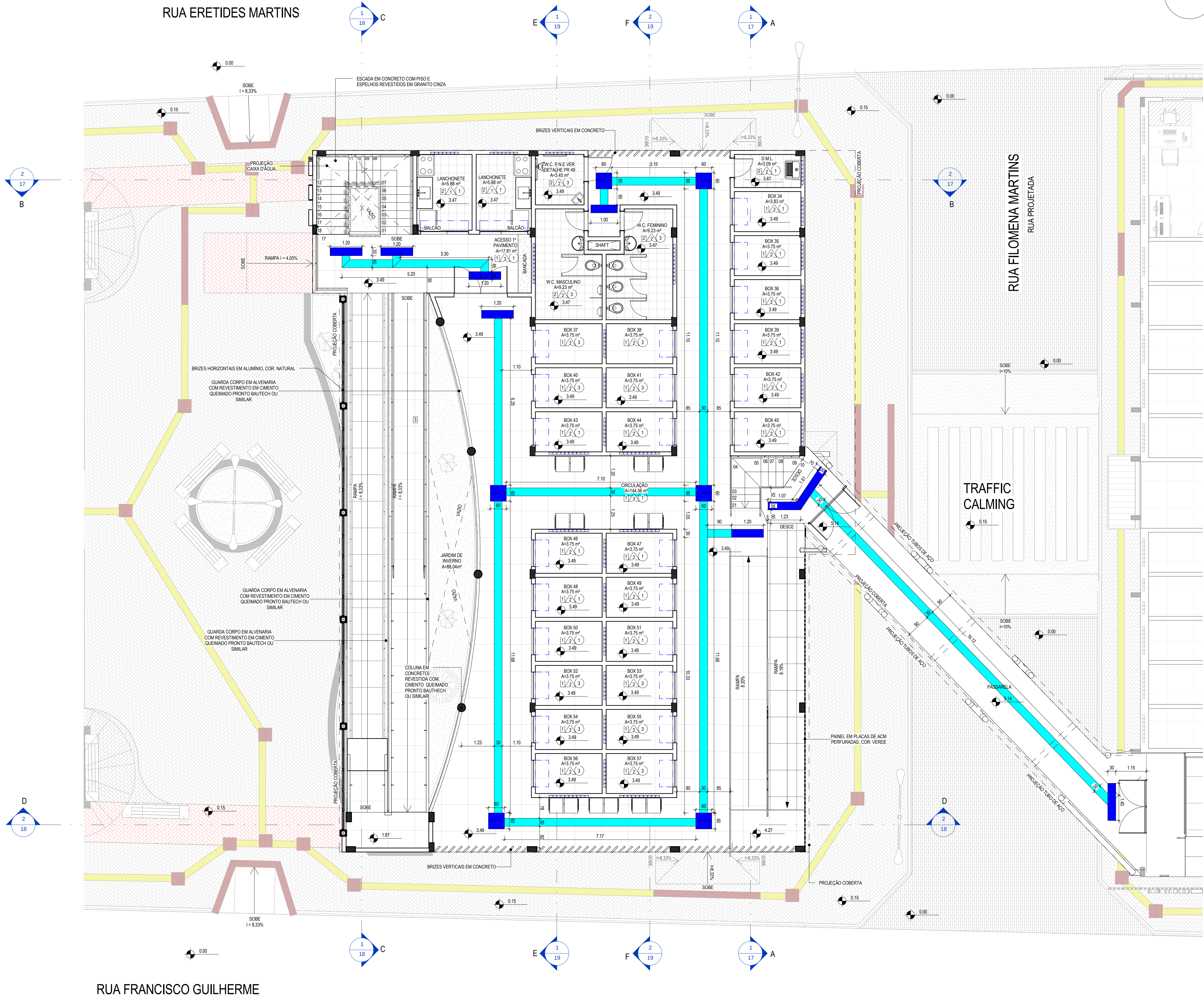
1 PLANTA DE ACESSIBILIDADE E PAGINAÇÃO - 1º PAVIMENTO ESCALA 1:75
