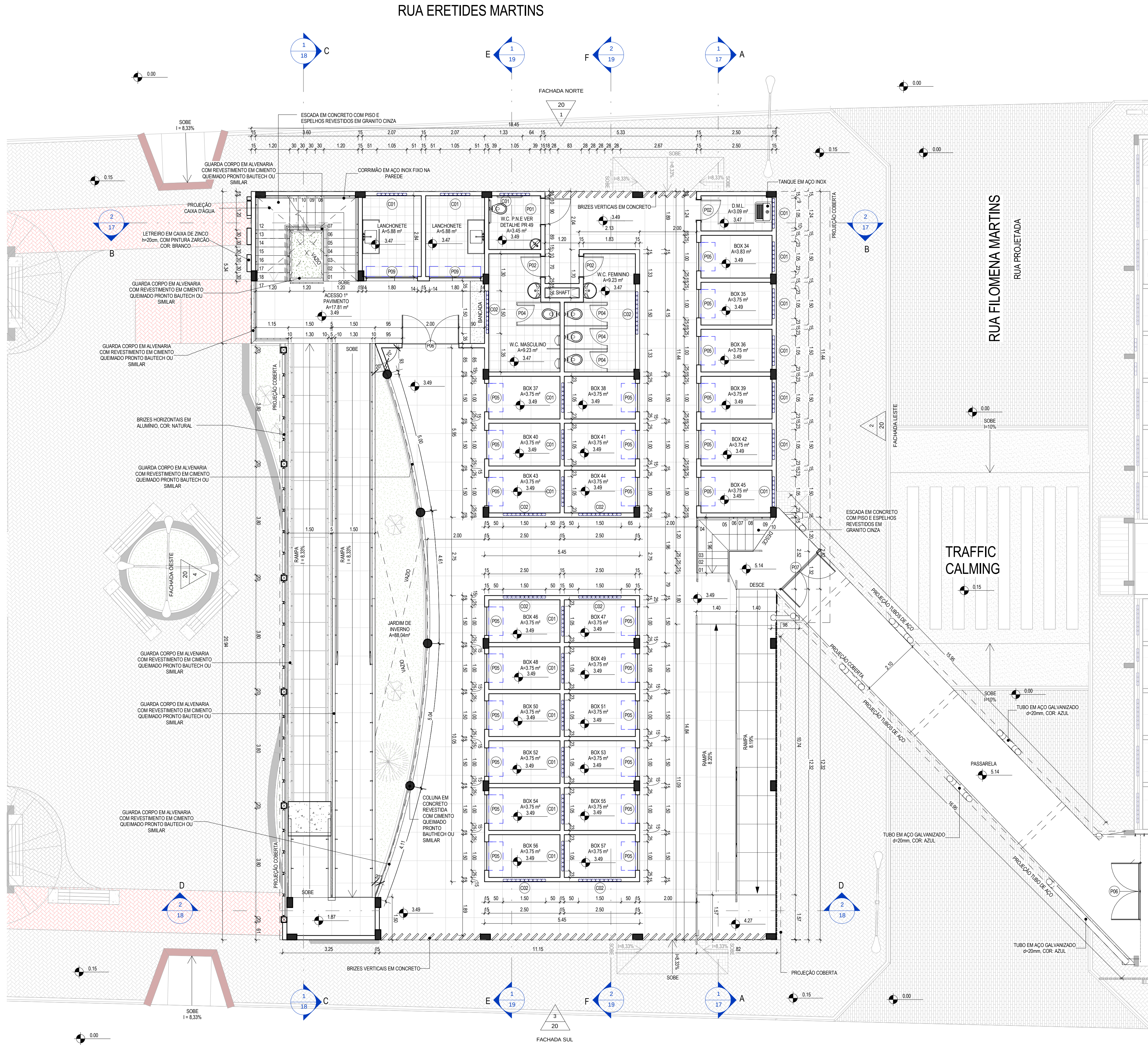
1 PLANTA TÉCNICA ANEXO - 1º PAVIMENTO ESCALA 1:75
