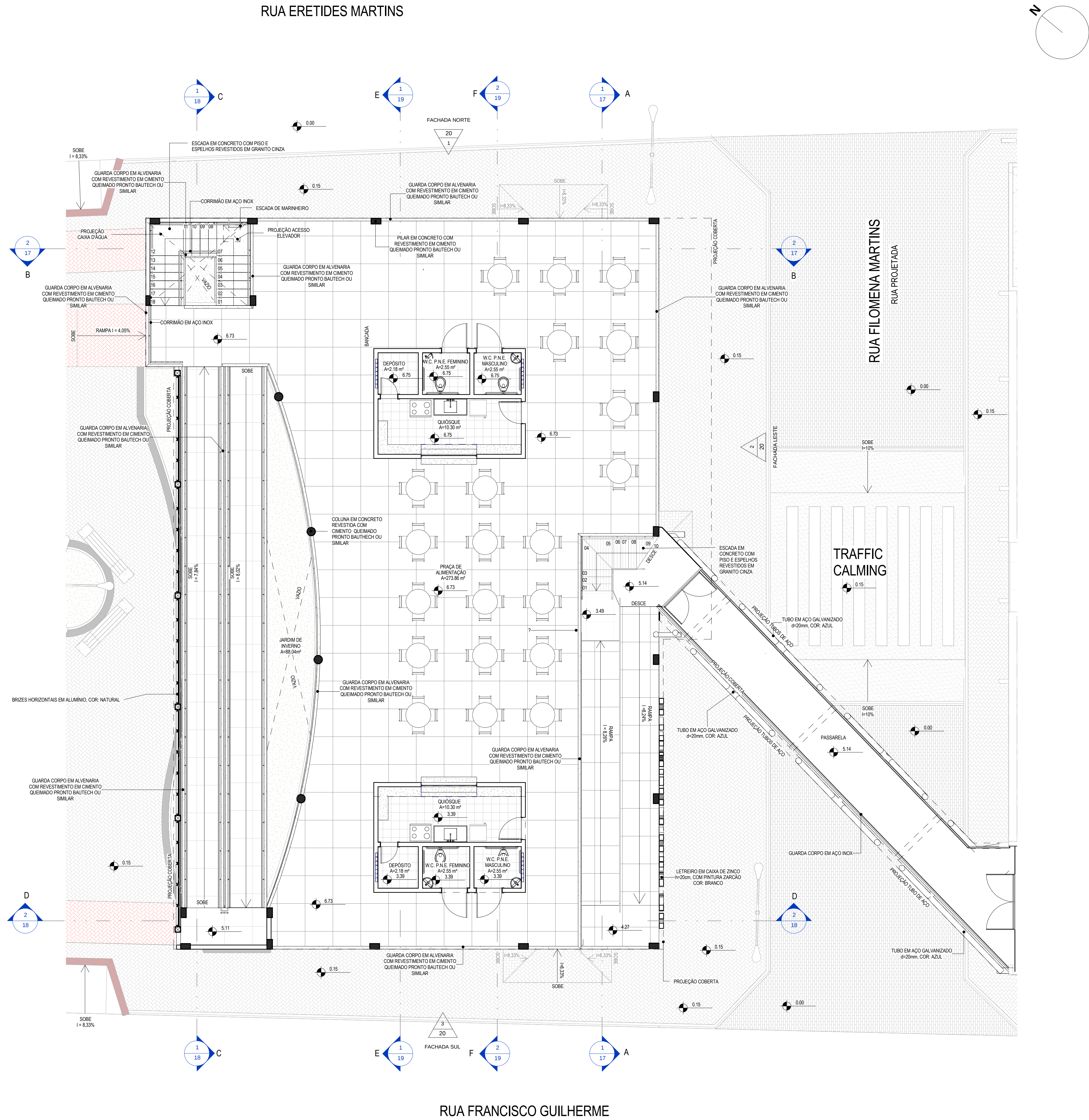
1 PLANTA DE LAYOUT - PRAÇA DE ALIMENTAÇÃO ESCALA 1:75
