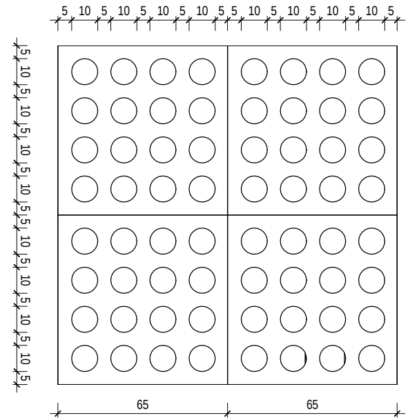
2 DETALHE PLACA DE ACM PERFURADA ESCALA 1:20
