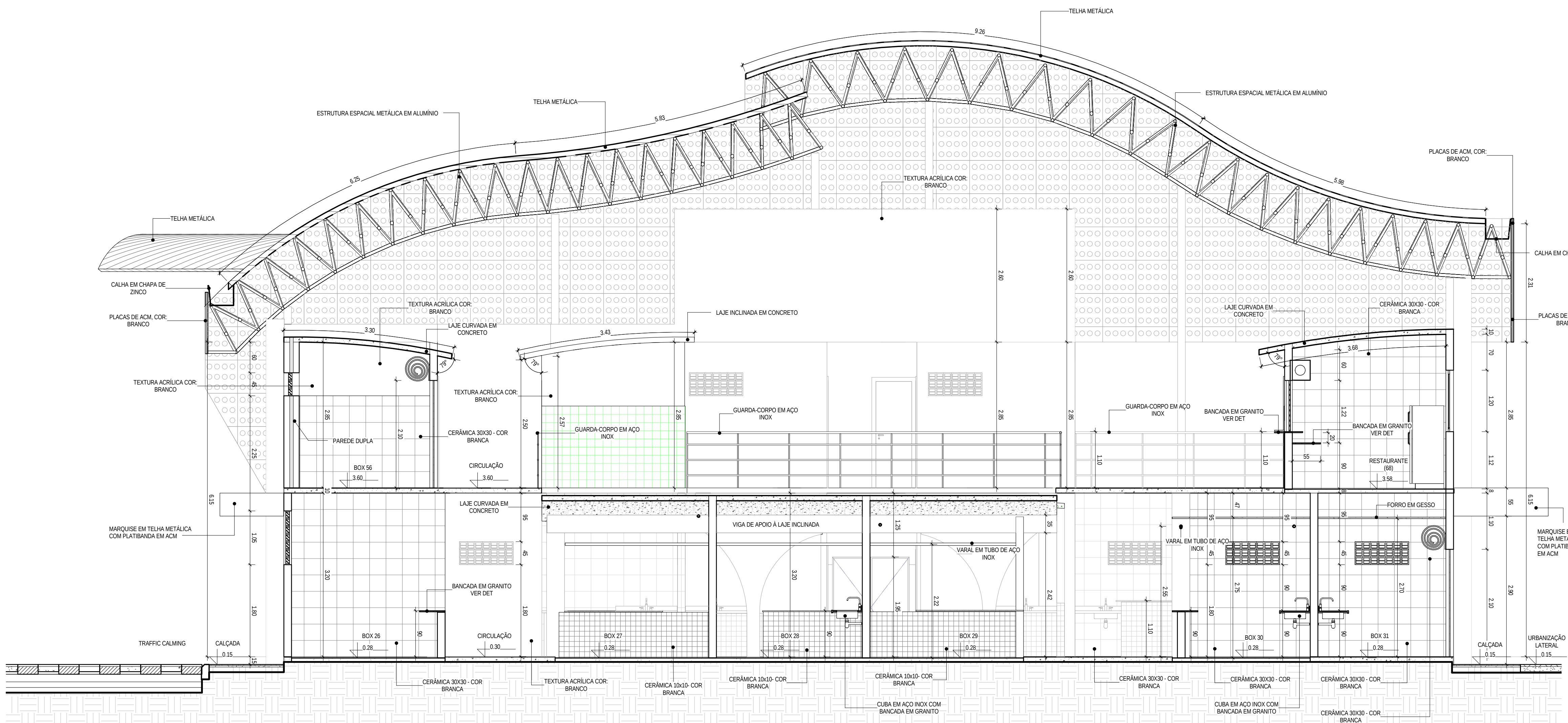
2 Corte F-F ESCALA 1:50
