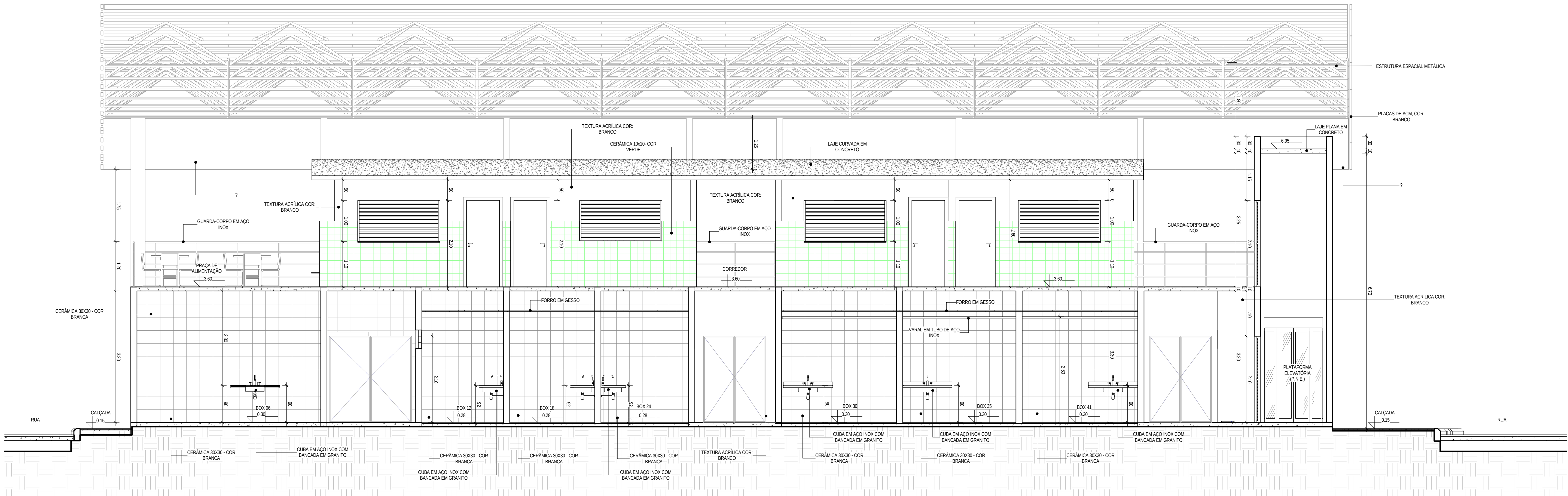
1 Corte E-E ESCALA 1:50
