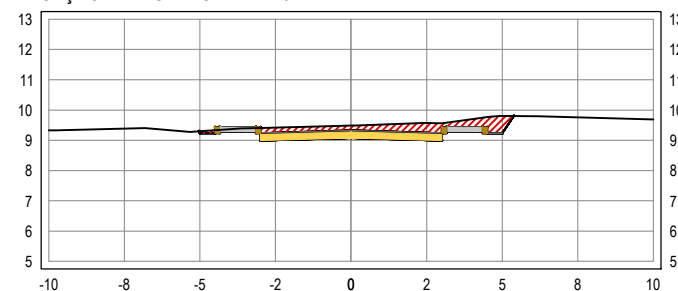
SEÇÃO TRANSVERSAL: 21+10
