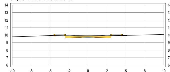
SEÇÃO TRANSVERSAL: 19+10
