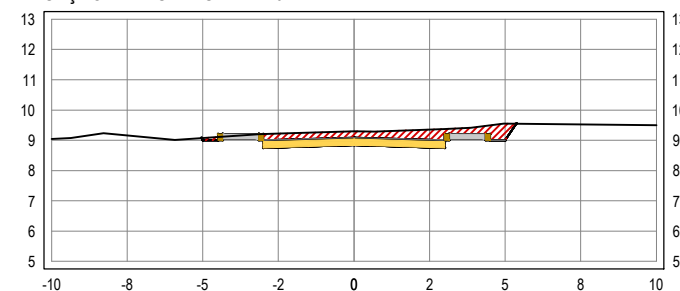
SEÇÃO TRANSVERSAL: 22+0
