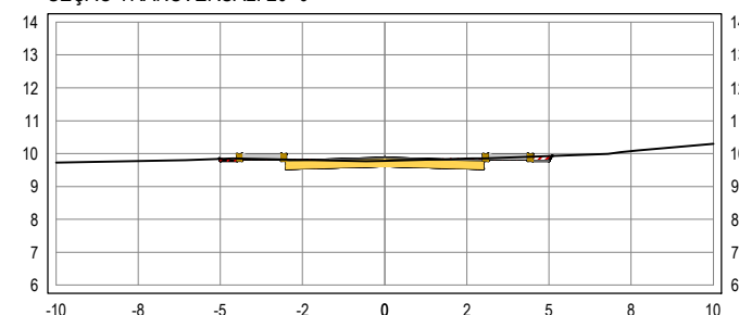
SEÇÃO TRANSVERSAL: 20+0
