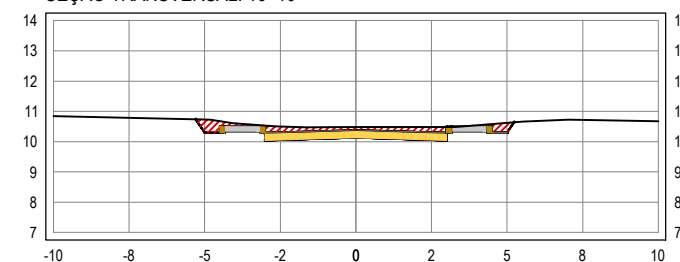
SEÇÃO TRANSVERSAL: 16+10
