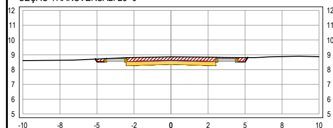
SEÇÃO TRANSVERSAL: 23+0
