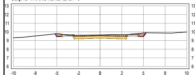
SEÇÃO TRANSVERSAL: 21+0
