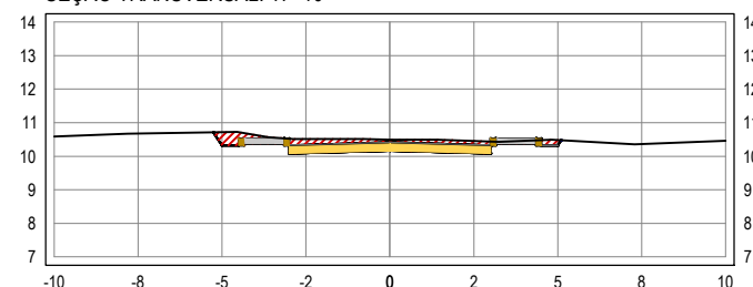
SEÇÃO TRANSVERSAL: 17+10
