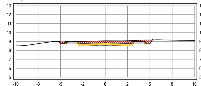
SEÇÃO TRANSVERSAL: 22+10
