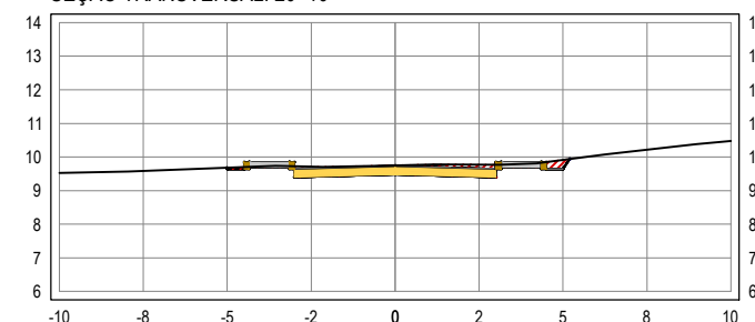
SEÇÃO TRANSVERSAL: 20+10
