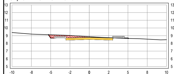
SEÇÃO TRANSVERSAL: 23+10
