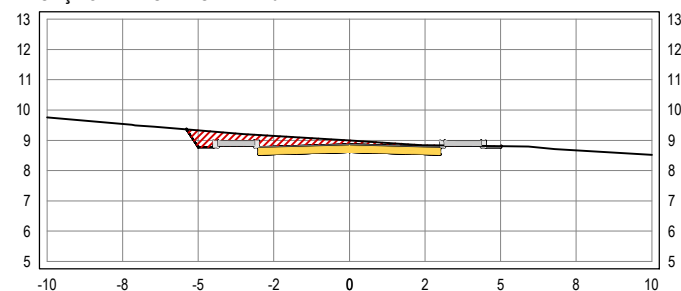
SEÇÃO TRANSVERSAL: 24+0
