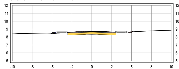
SEÇÃO TRANSVERSAL: 22+0
