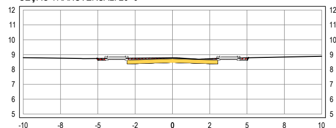
SEÇÃO TRANSVERSAL: 26+0
