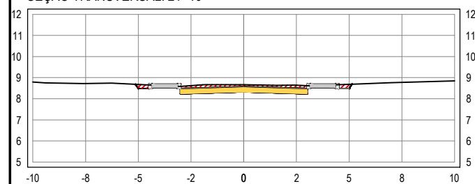
SEÇÃO TRANSVERSAL: 21+10
