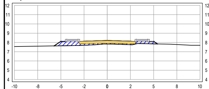
SEÇÃO TRANSVERSAL: 17+10
