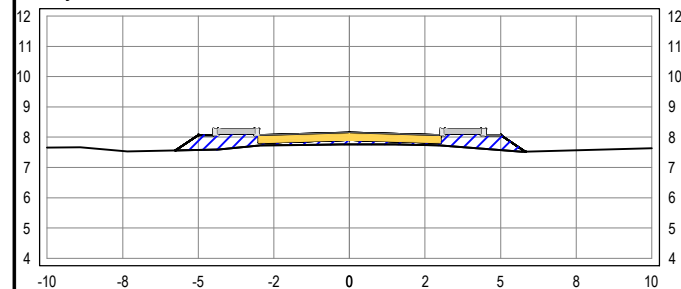
SEÇÃO TRANSVERSAL: 19+10
