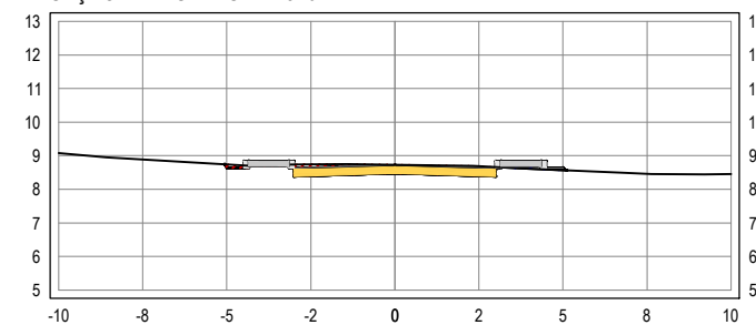
SEÇÃO TRANSVERSAL: 23+0
