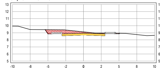
SEÇÃO TRANSVERSAL: 24+10
