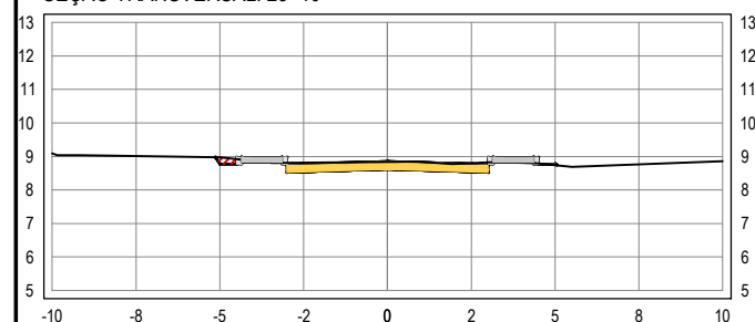
SEÇÃO TRANSVERSAL: 25+10
