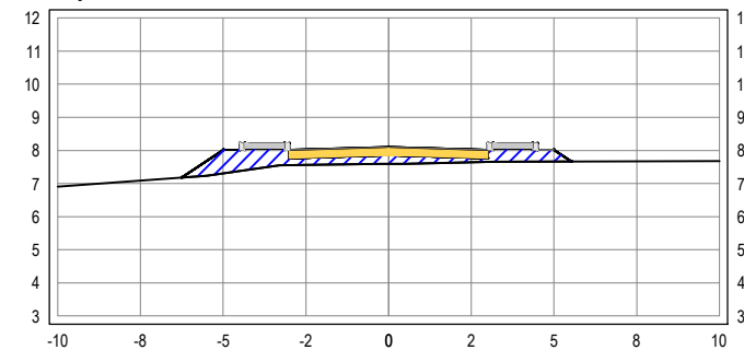
SEÇÃO TRANSVERSAL: 19+0
