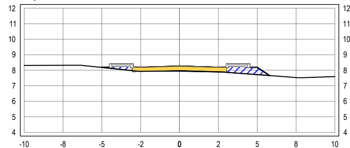
SEÇÃO TRANSVERSAL: 20+0
