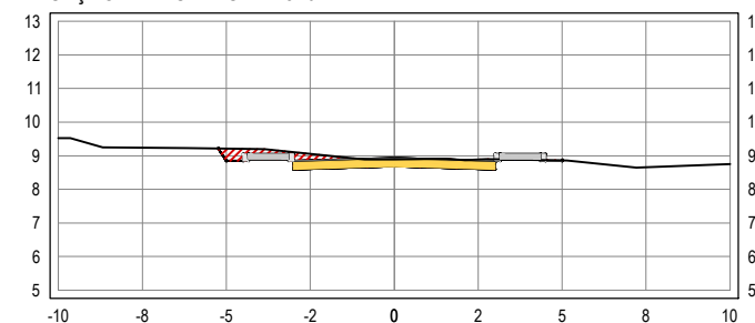
SEÇÃO TRANSVERSAL: 25+0
