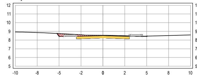
SEÇÃO TRANSVERSAL: 21+0
