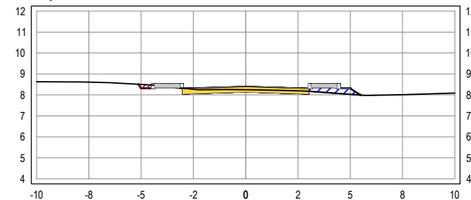
SEÇÃO TRANSVERSAL: 20+10
