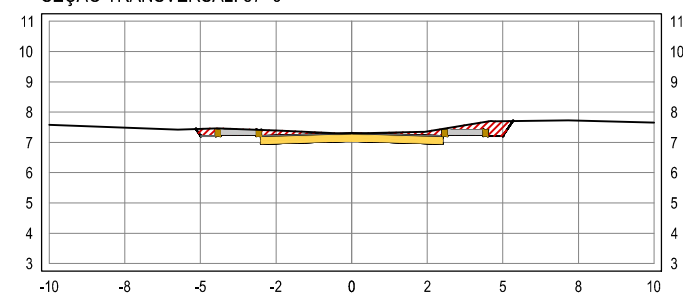
SEÇÃO TRANSVERSAL: 57+9
