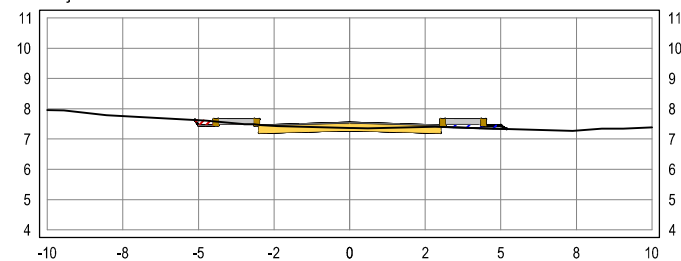
SEÇÃO TRANSVERSAL: 55+0
