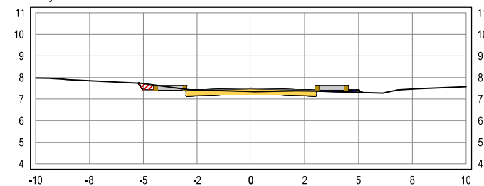
SEÇÃO TRANSVERSAL: 55+10
