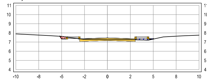
SEÇÃO TRANSVERSAL: 56+0
