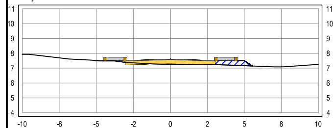
SEÇÃO TRANSVERSAL: 54+10
