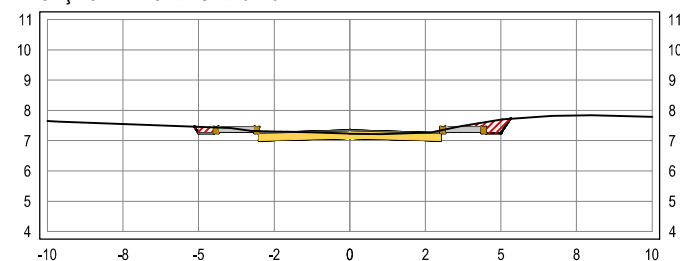
SEÇÃO TRANSVERSAL: 57+0
