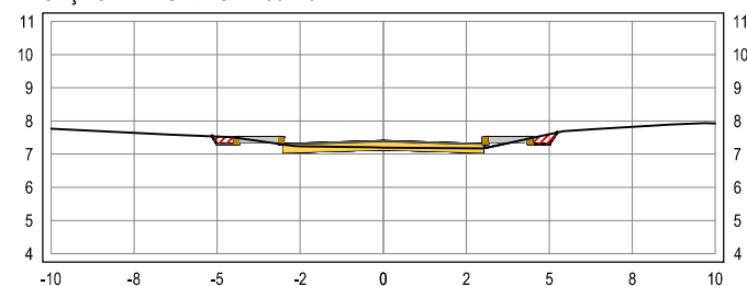
SEÇÃO TRANSVERSAL: 56+10
