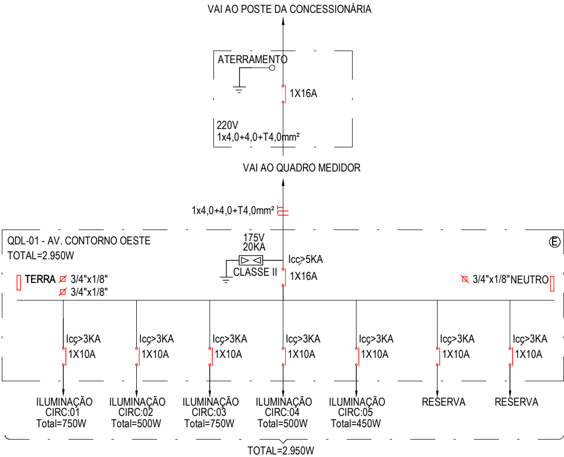
2 DIAGRAMA UNIFILAR - QDL-01 ESCALA 1 : 125
