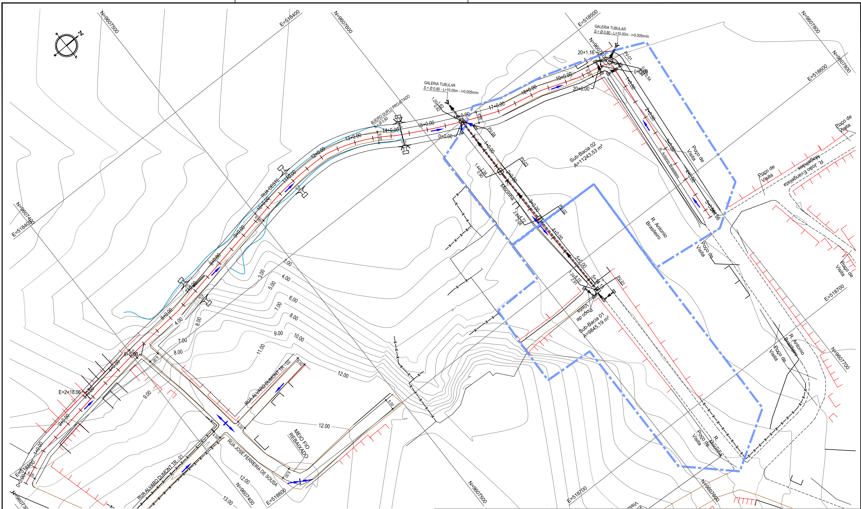
01 PLANTA BAIXA 01 ESCALA: 1/1500
