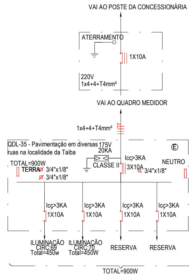
3 DIAGRAMA UNIFILAR - QDL-35 ESCALA 1 : 125
