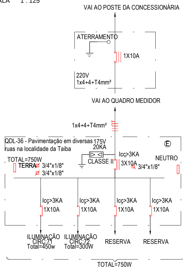
4 DIAGRAMA UNIFILAR - QDL-36 ESCALA 1 : 125
