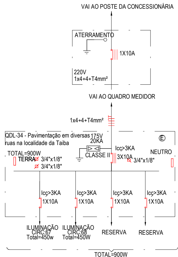
2 DIAGRAMA UNIFILAR - QDL-34 ESCALA 1 : 125
