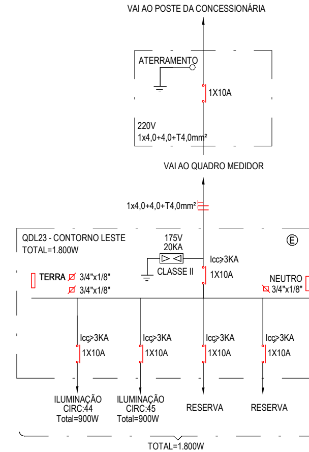
3 Diagrama Unifilar - QDL 23 ESCALA 1 : 125
