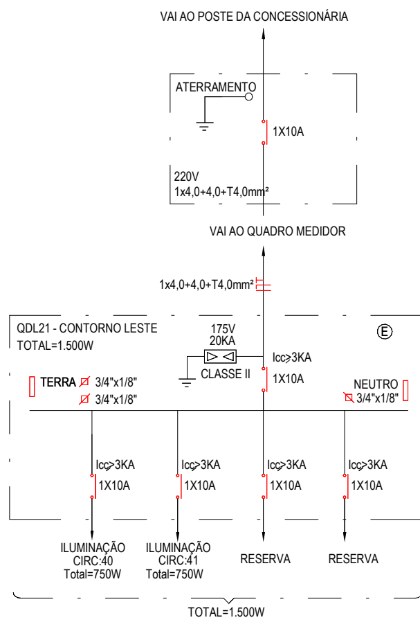
1 Diagrama Unifilar - QDL 21 ESCALA 1 : 125
