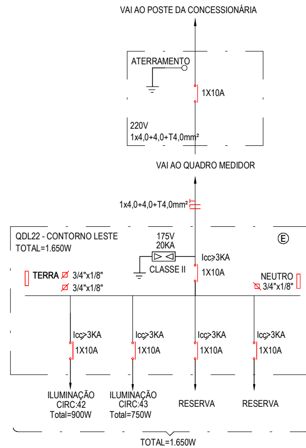
2 Diagrama Unifilar - QDL 22 ESCALA 1 : 125
