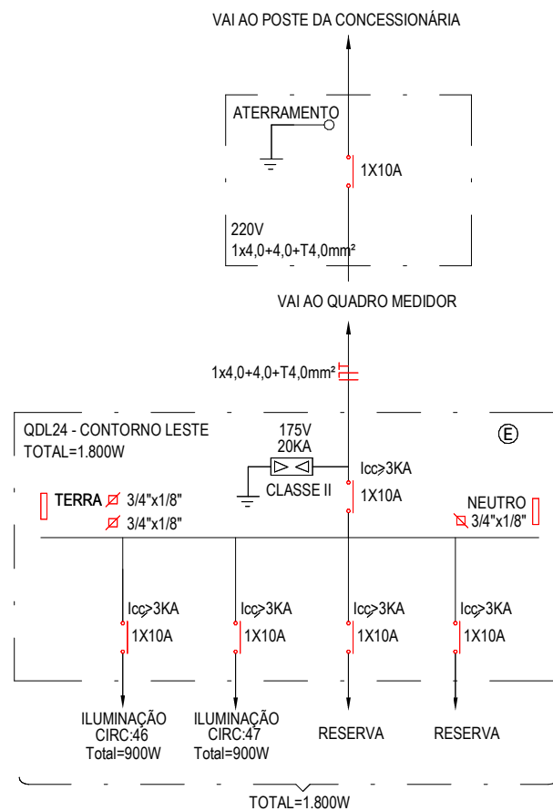
4 Diagrama Unifilar - QDL 24 ESCALA 1 : 125
