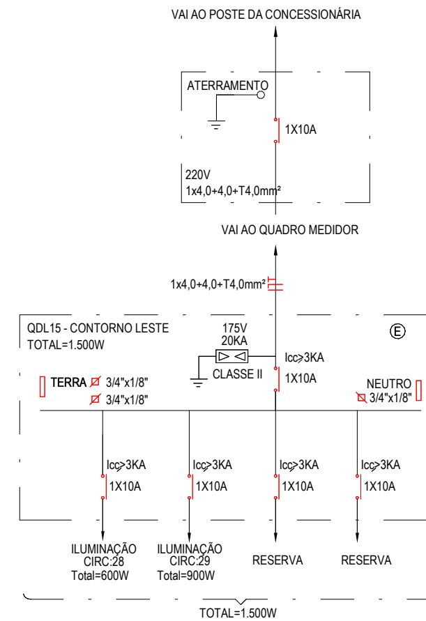
3 Diagrama Unifilar - QDL 15 ESCALA 1 : 125
