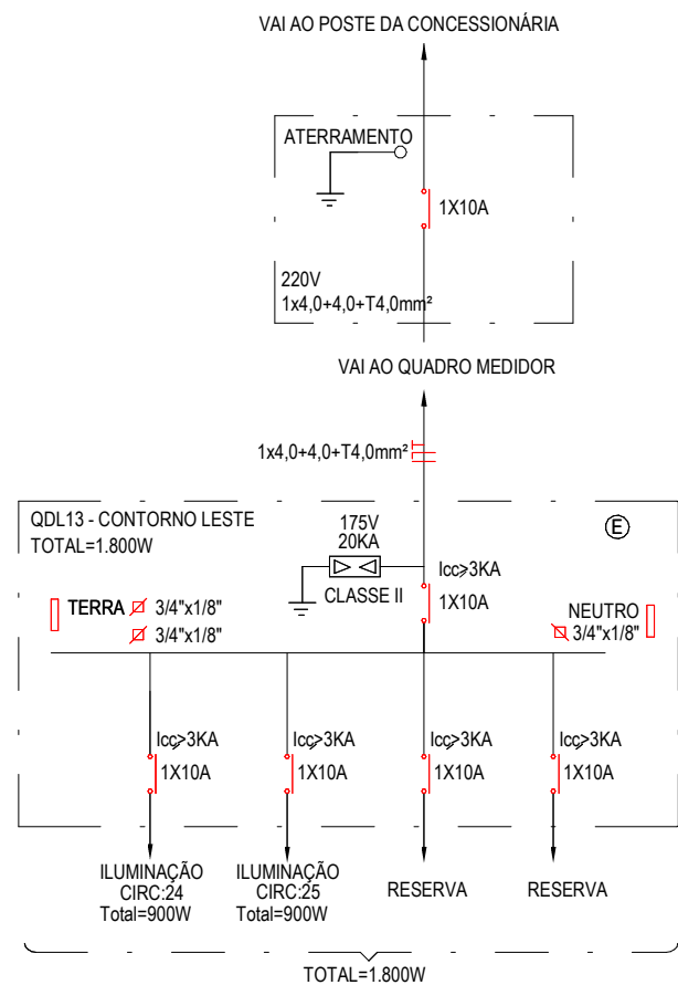
1 Diagrama Unifilar - QDL 13 ESCALA 1 : 125
