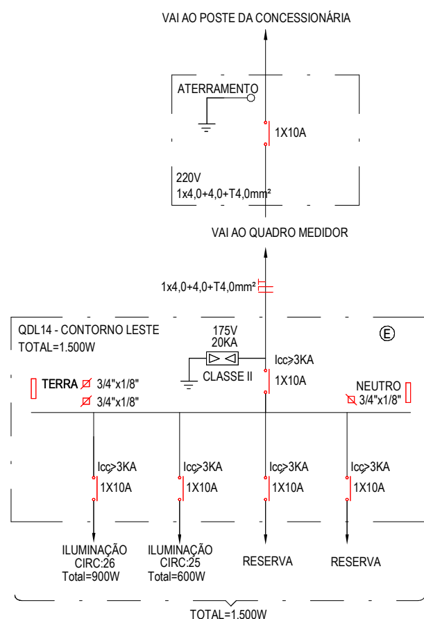
2 Diagrama Unifilar - QDL 14 ESCALA 1 : 125
