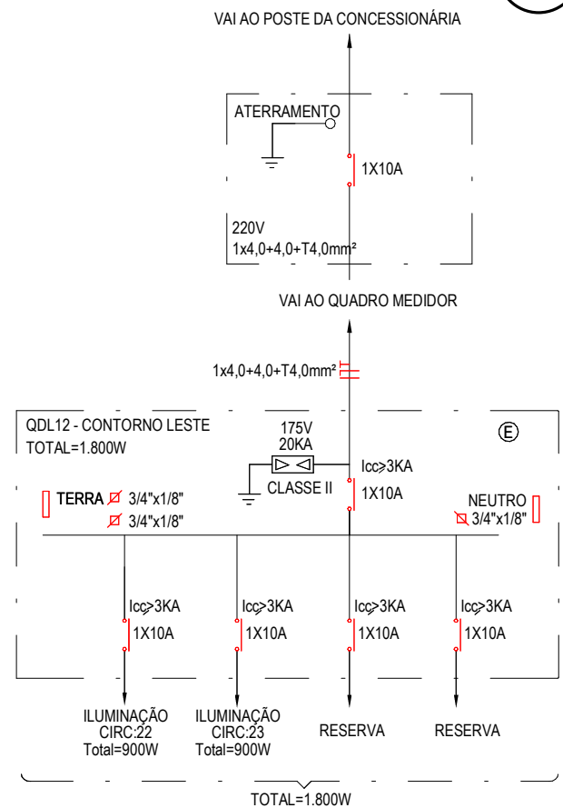
4 Diagrama Unifilar - QDL 12 ESCALA 1 : 125
