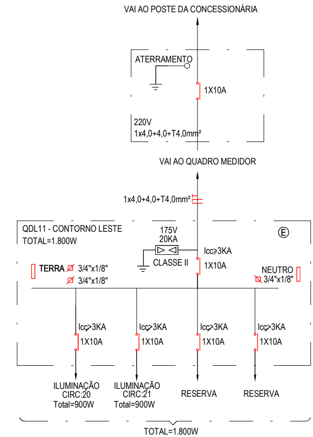
3 Diagrama Unifilar - QDL 11 ESCALA 1 : 125
