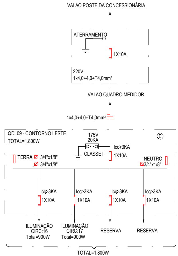
1 Diagrama Unifilar - QDL 09 ESCALA 1 : 125
