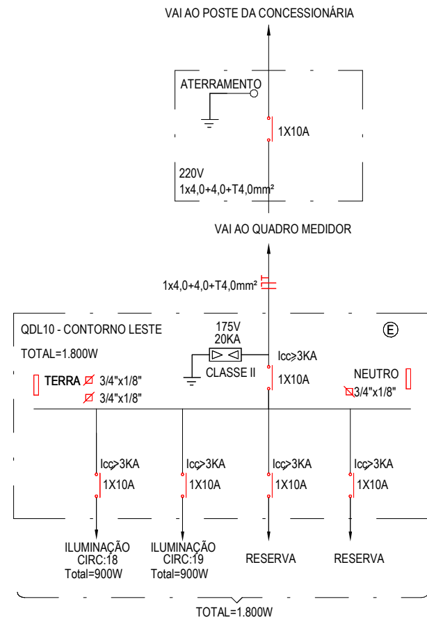
2 Diagrama Unifilar - QDL 10 ESCALA 1 : 125
