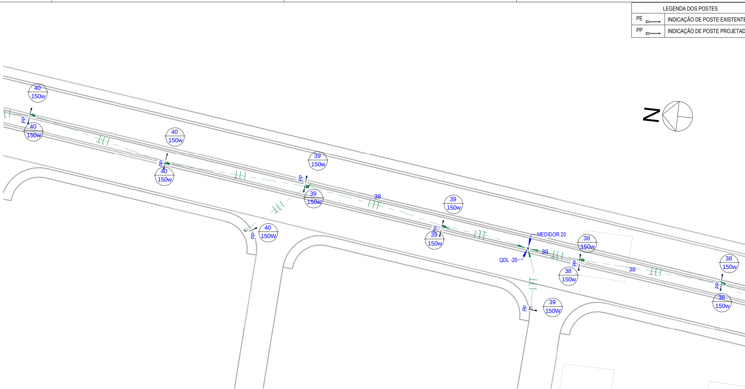
1 Planta Baixa - Iluminação - Trecho 18 ESCALA 1 : 500
