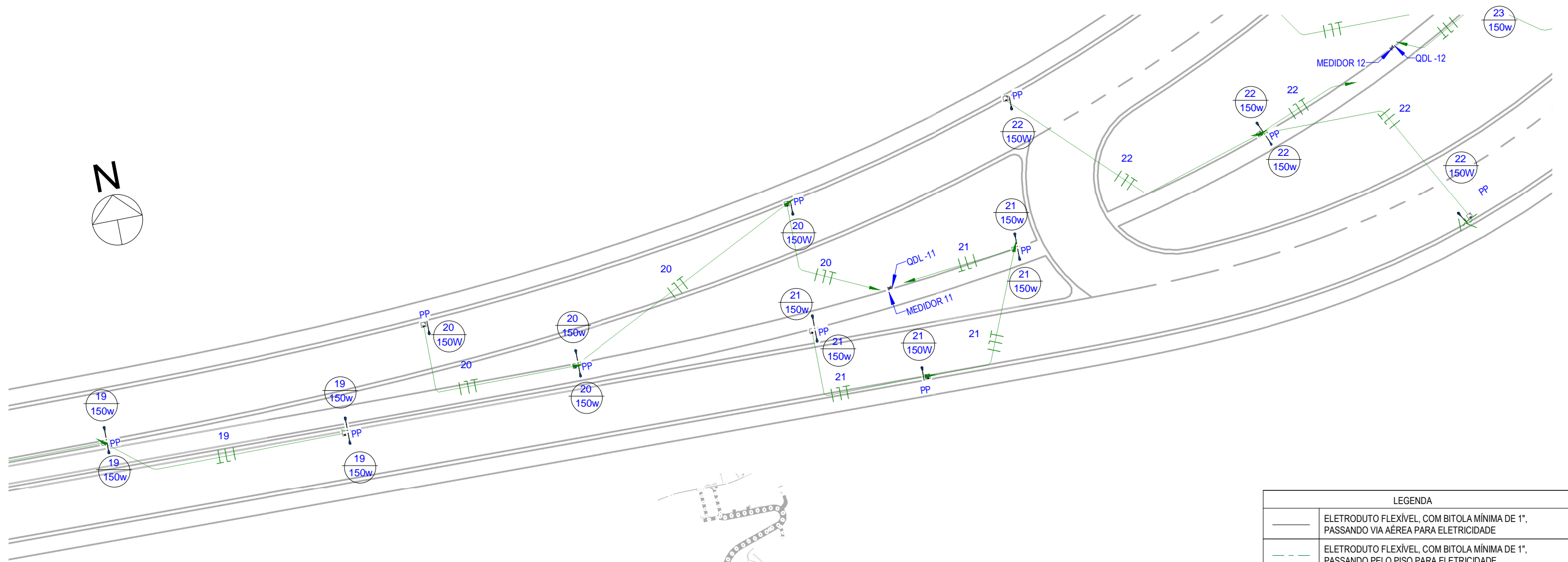
1 Planta Baixa - Iluminação - Trecho 11 ESCALA 1 : 500
